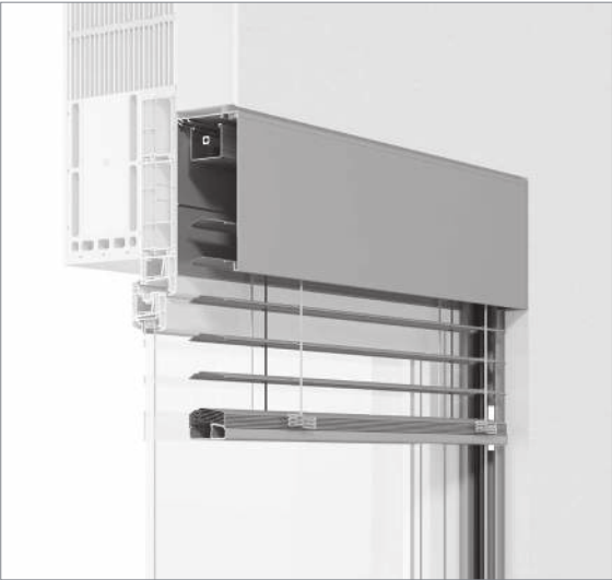
EXPRESS B - sichtbare Blende
