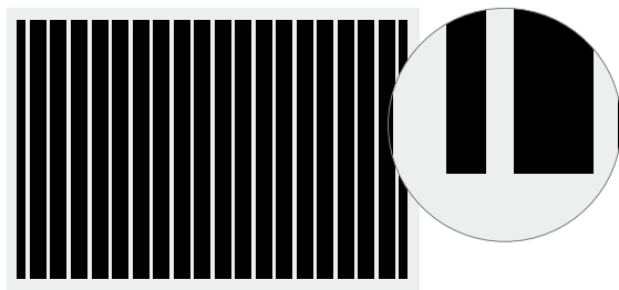
NEU. Motiv 470 (ET 450) Füllung mit verzinkten Quadratrohrstäben 30 x 30 x 1 mm, Lüftungsquerschnitt 77%
