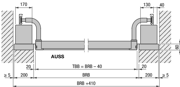
Horizontalschnitt
