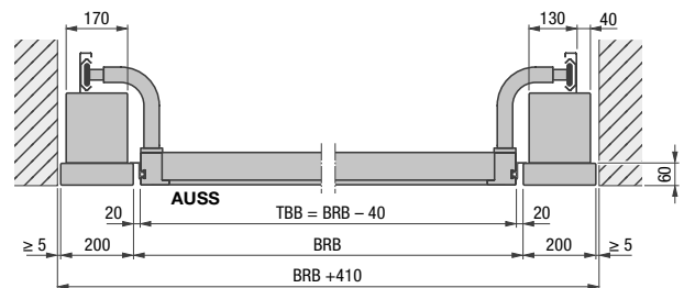
Horizontalschnitt
