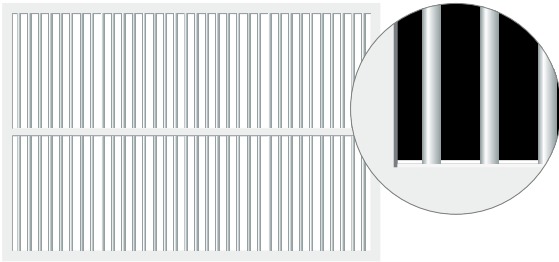
Motiv 470 Füllung mit Aluminium-Stäben 20 x 20 x 2 mm, Lüftungsquerschnitt 80%
