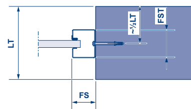
Platzbedarf Führungsschiene FS60x75
