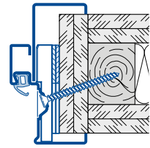
Diagonalbefestigung Montagewand F90B C Typ 1
