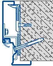
Diagonalbefestigung Porenbeton bis MW 450 D Typ 1
