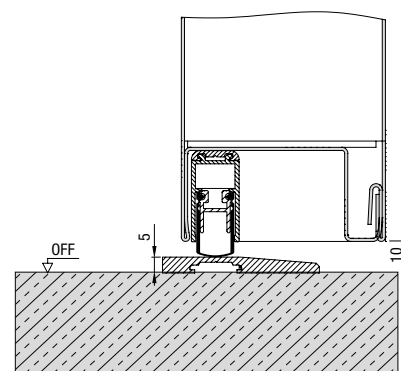
3 mit Dichtung und Höckerschwelle
