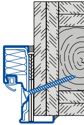
Diagonalbefestigung Montagewand F90B B Typ 1
