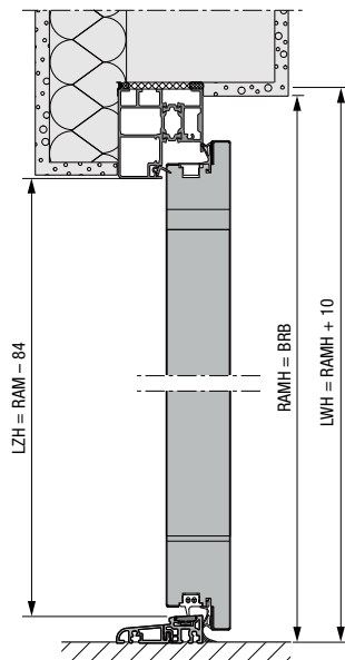
Vertikalschnitt
