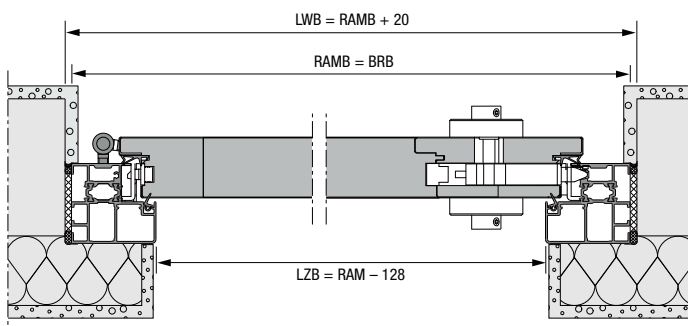
Horizontalschnitt
