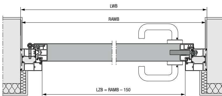
Zargenvarianten
