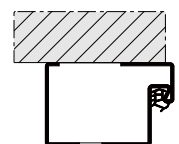
Blockzarge für Montage auf der Wand (Profil 006) (geprüft auf der Band- gegensseite)
