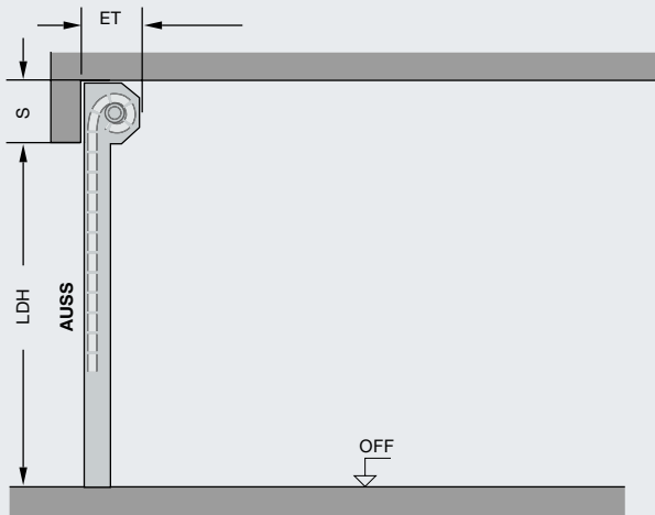
Vertikalschnitt
