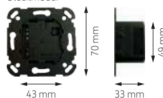
Steckmodul
